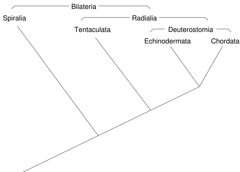
Abbildung 2: Die phylogenetische Verwandtschaft innerhalb der Bilateria unter Betonung der Eingliederung der Echinodermata, kombiniert nach [1] und HEJNOL in [2]
