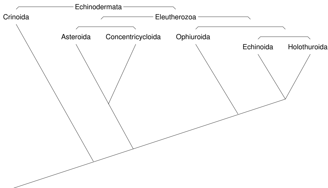
Abbildung 3: Hypothetisches Kladogramm der Echinodermata, aus [12], verändert
