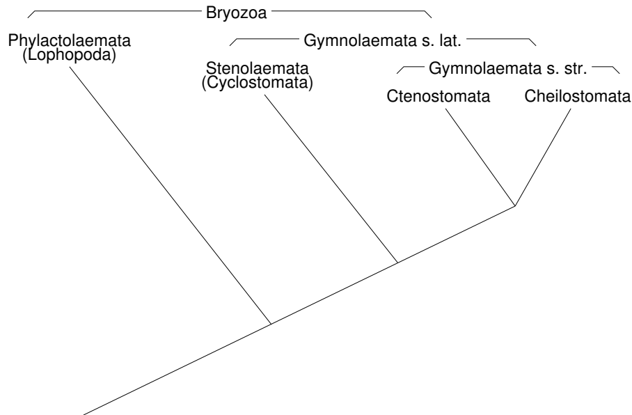
Abbildung 4: Diagramm der phylogenetischen Verwandtschaft innerhalb der Bryozoa, kombiniert nach [7] und [12]
