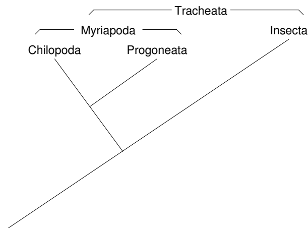
Abbildung 5: Die phylogenetische Verwandtschaft innerhalb der Tracheata aus Sicht der Myriapoda-Hypothese, aus [1]
