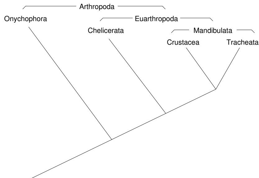
Abbildung 1: Diagramm der phylogenetischen Verwandtschaft innerhalb der Arthropoda, aus [1]
