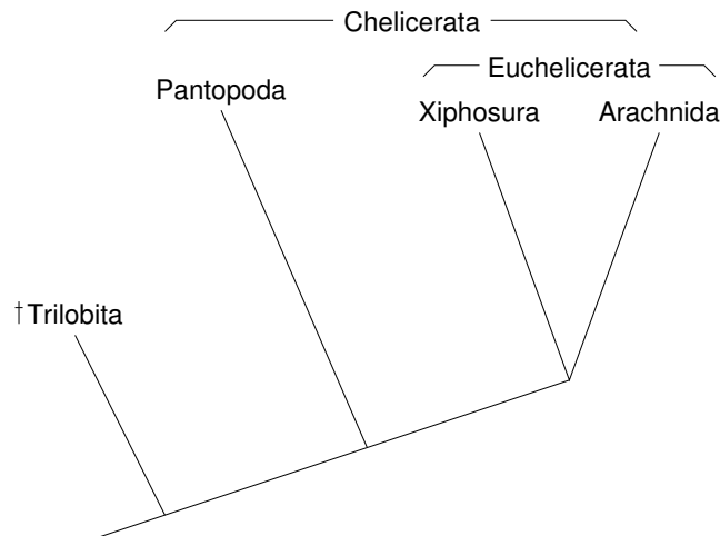
Abbildung 4: Diagramm der phylogenetischen Verwandtschaft innerhalb der Chelicerata, ergänzt um die †Trilobita, aus [1], verändert nach [2]
